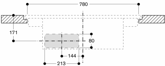
Vooraanzicht - meubeluitsnede voor kanaalloze recirculatie; vlak geïntegreerde inbouw
