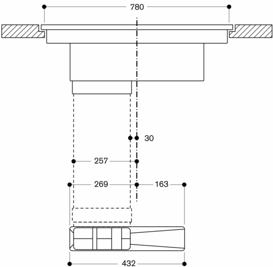
Frontaanzicht van CV 282 met kanaal-luchtrecirculatie
