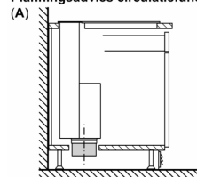
A: Buitenwand – U-waarde \leq 0,5 \text{ W/(m}^2\text{K)}
