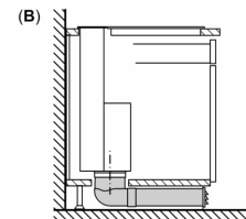
B: Buitenwand – U-waarde > 0,5 \text{ W/(m}^2\text{K)}
