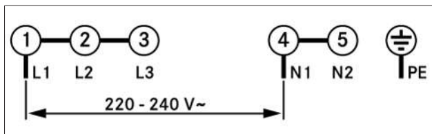
Afb. 9.24 Aansluitschema 1-faseaansluiting
