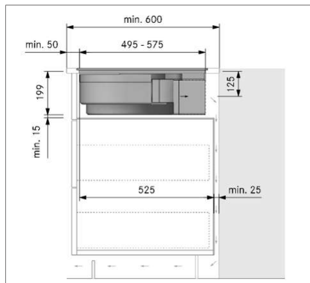
Afb. 9.13 Inbouwmaten bij recirculatie - montagevariant B, werkbladdiepte 600 mm
