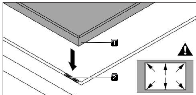
Afb. 9.18 Positionering van de vulplaatjes
