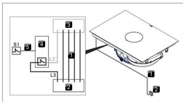
Afb. 9.22 Aansluitschema met extern schakelcontact
