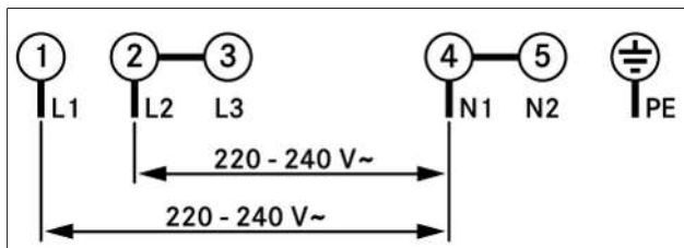
Afb. 9.25 Aansluitschema 2-faseaansluiting
