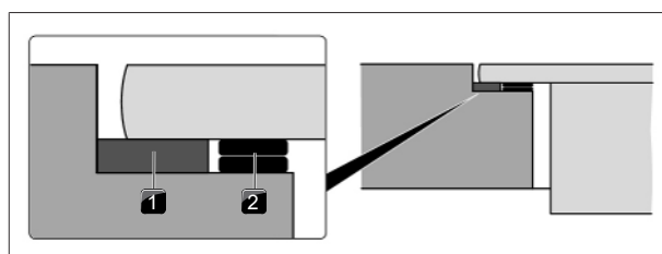
Afb. 9.19 Vulplaatjes
