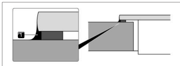
Afb. 9.30 Siliconenkit bij opbouwmontage
