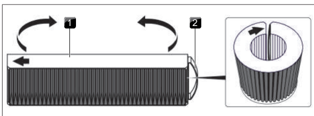
Afb. 7.5 Geurfilter
