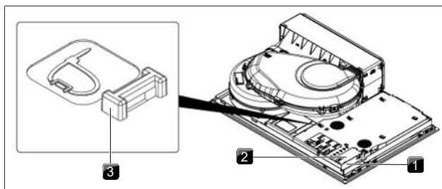
Afb. 9.26 Elektrische aansluitingen van het kookveld
