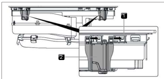
Afb. 9.16 Montageklemmen aanbrengen
