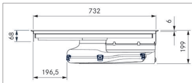
Afb. 3.2 Apparaatafmetingen vooraanzicht
