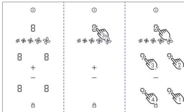
Afb. 9.27 Display dealer- en servicemenu oproepen
