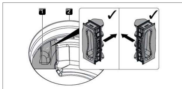
Afb. 7.8 Filtervervangingsklep plaatsen
