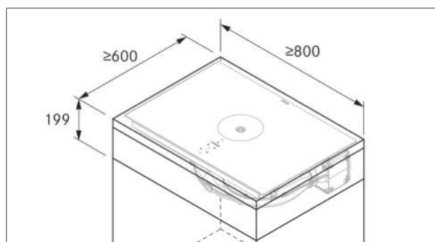
Afb. 9.2 Minimale meubelafmetingen
