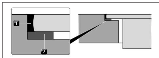
Afb. 9.15 Afdichtingsband bij vlainbouw
