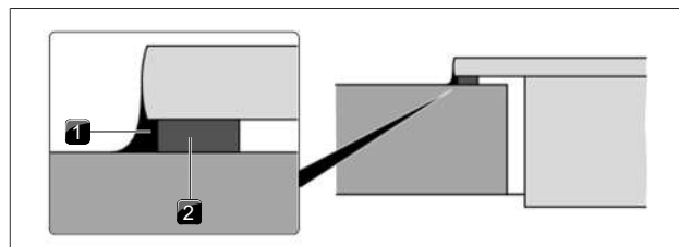
Afb. 9.14 Afdichtingsband bij opbouwmontage
