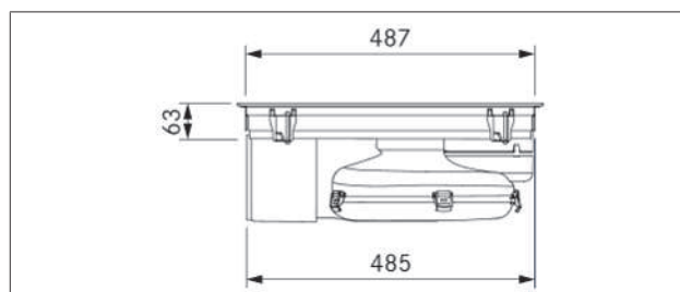
Afb. 3.3 Apparaatafmetingen zijaanzicht
