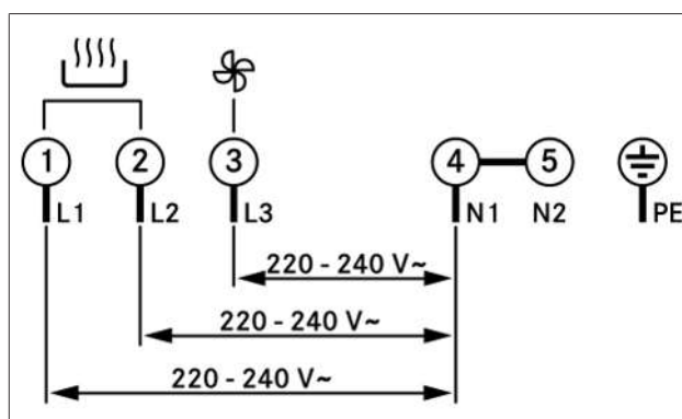
Afb. 9.23 Aansluitschema 3-faseaansluiting
