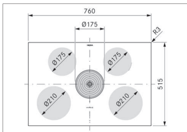
Afb. 3.1 Apparaatafmetingen bovenaanzicht
