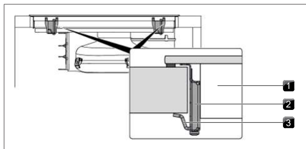
Afb. 9.20 Centrale bevestiging kookveld
