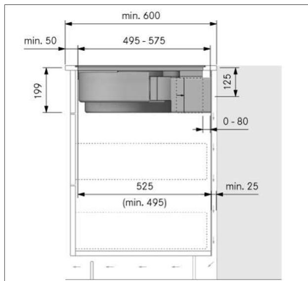
Afb. 9.10 Inbouwmaten bij recirculatie, montagevariant A
