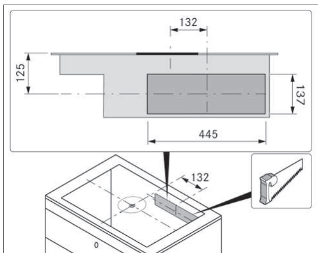
Afb. 9.8 Achterwanduitsparing
