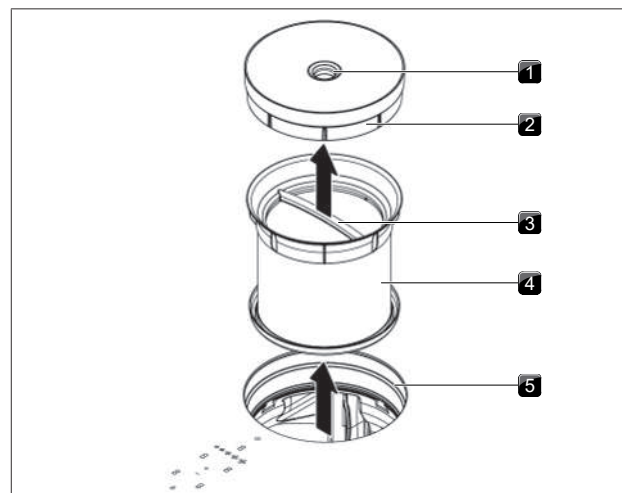
Afb. 7.1 Demonteren van de onderdelen
