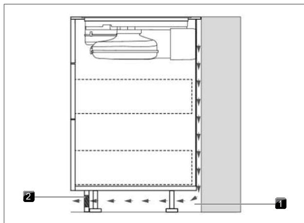
Afb. 9.7 Terugstroomopening in plintgedeelte
