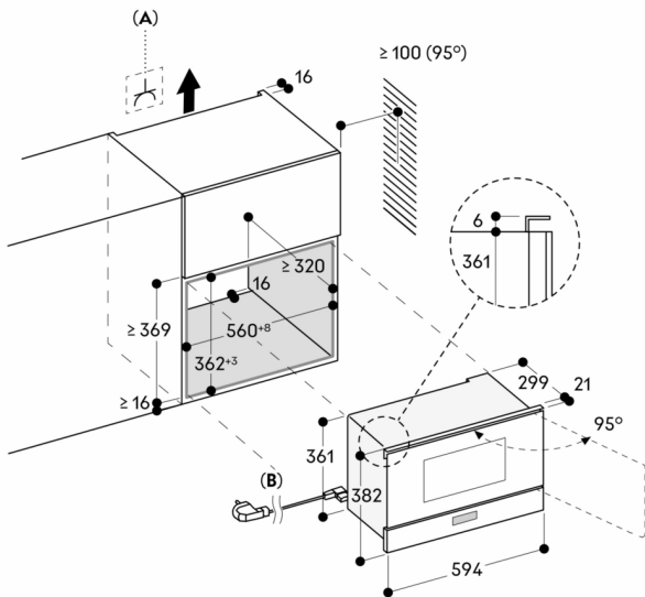
A: Toegankelijke elektrische aansluiting B: Kabel met of zonder stekker, afhankelijk van het land Afmeting in mm
