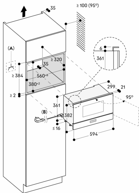
A: Toegankelijke elektrische aansluiting B: Kabel met of zonder stekker, afhankelijk van het land Afmeting in mm
