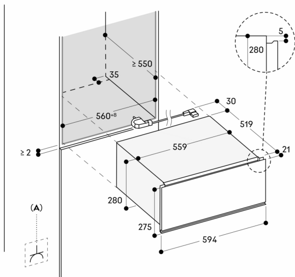
A: Toegankelijke elektrische aansluiting Afmeting in mm
