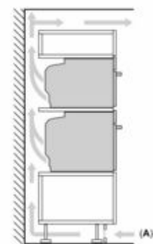
Inbouw van twee apparaten boven elkaar Luchtverversing
