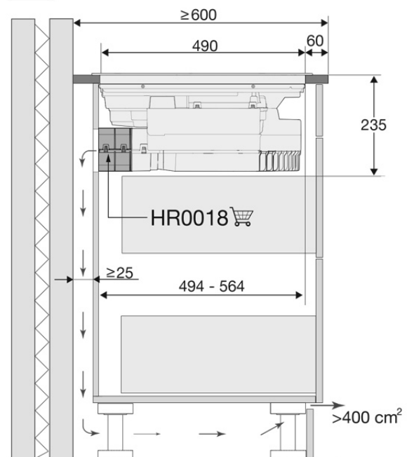
Recirculatie door achterwand
