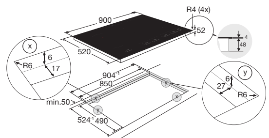
Vlak inbouw / Flush installation
