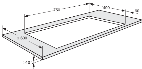
Opbouw / Top installation
