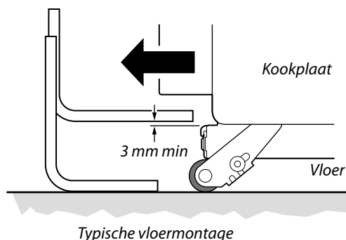
Stabiliteitsbeugel
