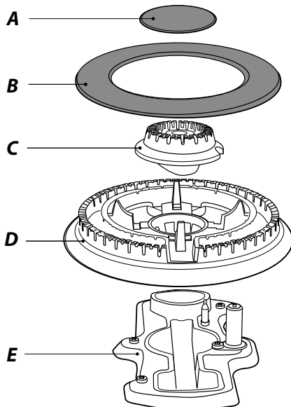
A – Binnenbranderkap, B – Buitenbranderkap, C – Binnenbranderkop, D – Buitenbranderkop, E – Wokbranderbasis
