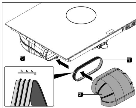
Afb. 11.24 Aansluiting op het kanaalsysteem
