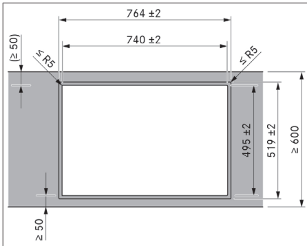
Afb. 11.5 Uitsparingsafmetingen in geval van vlakinbouw
