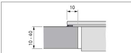
Afb. 11.8 Oplegmaat voor opbouwmontage
