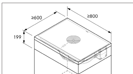
Afb. 11.4 Minimale meubelafmetingen
