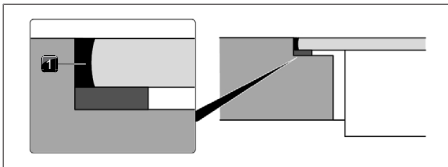
Afb. 11.36 Siliconenkit bij vlakinbouw
