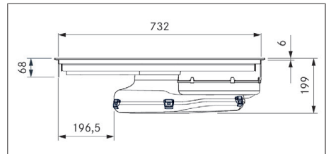
Afb. 3.2 PURA2/R apparaatafmetingen vooraanzicht
