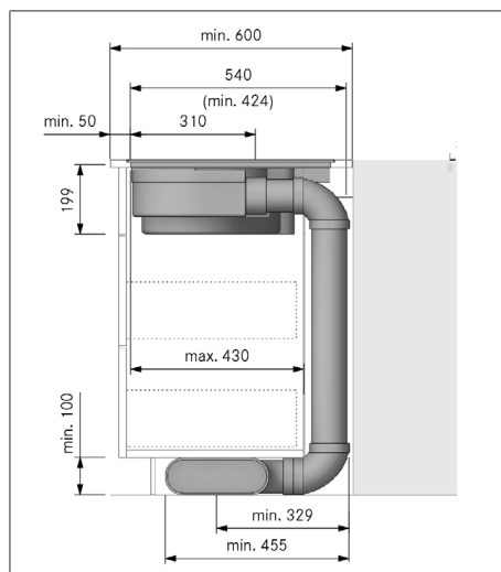
Afb. 11.9 Inbouwmaten luchtafvoer, werkbladdiepte 600 mm
