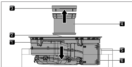
Afb. 11.20 Centrale plaatsing kookveld
