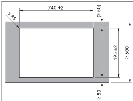
Afb. 11.7 Uitsparingsafmetingen in geval van opbouwmontage
