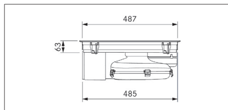
Afb. 3.6 PURU2/R apparaatafmetingen zijaanzicht
