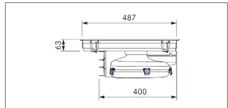
Afb. 3.3 PURA2/R apparaatafmetingen zij aanzicht
