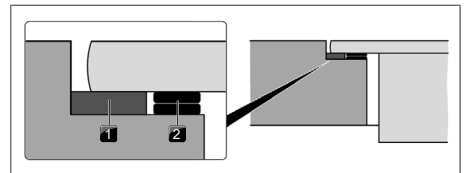
Afb. 11.22 Vulplaatjes
