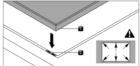
Afb. 11.21 Positionering van de vulplaatjes
