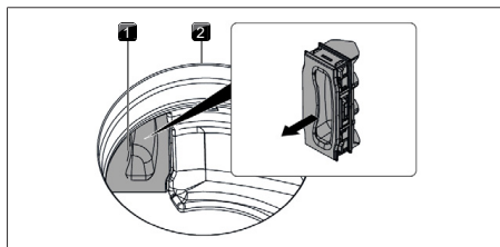
Afb. 9.4 Filtervervangingsklep verwijderen
