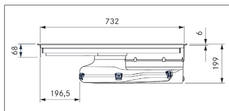
Afb. 3.5 PURU2/R apparaatafmetingen vooraanzicht
