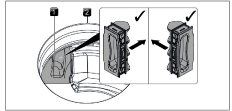
Afb. 9.10 Filtervervangingsklep plaatsen
