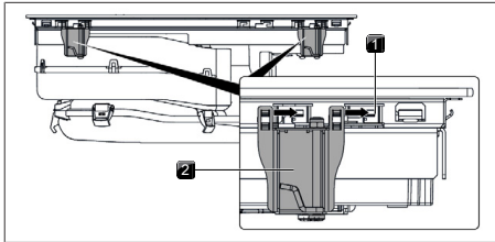
Afb. 11.19 Montageklemmen aanbrengen
