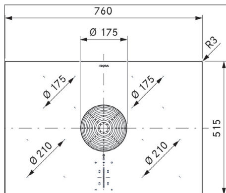
Afb. 3.4 PURU2/R apparaatafmetingen bovenaanzicht
