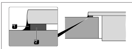
Afb. 11.17 Afdichtingsband bij opbouwmontage
