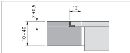
Afb. 11.6 Voegmaat voor vlakinbouw
