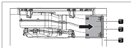
Afb. 11.25 Aansluiting op de achterwand
