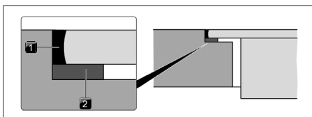
Afb. 11.18 Afdichtingsband bij vlakinbouw
