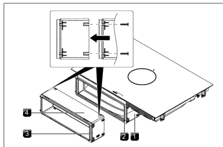
Afb. 11.15 Verlenging telescopisch kanaal
