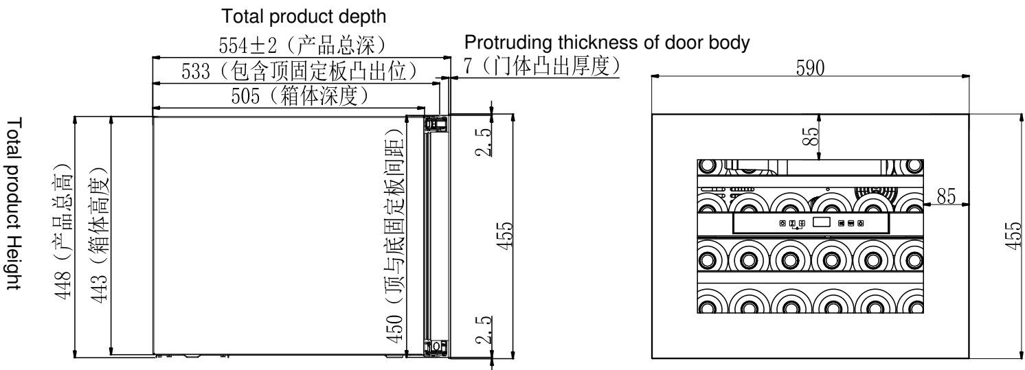
侧视图
