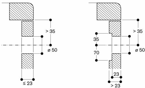
Montage bedieningsknop, inbouw met zichtbare rand
