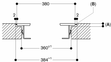
Doorsnede in de lengte
