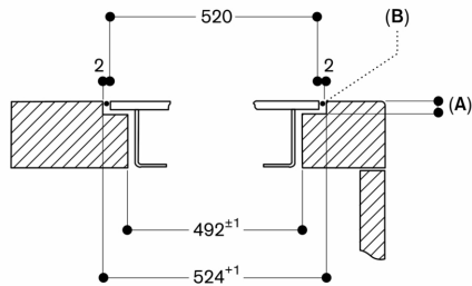
Dwarsdoorsnede
