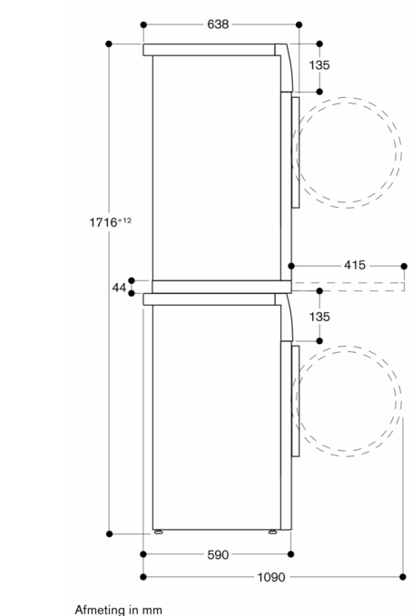
Zijaanzicht van WT 260 boven WM 260 met aansluitset-accessoire
